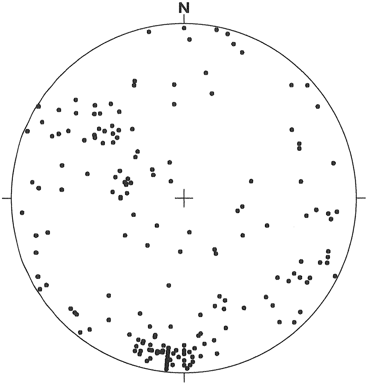
Lower hemisphere - Trennflächen Niernberg - Aufschlüsse - N=208
