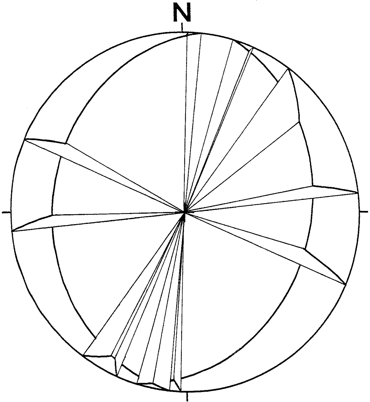
Lower hemisphere - Großkreisdarstellung Niemberg N=7
